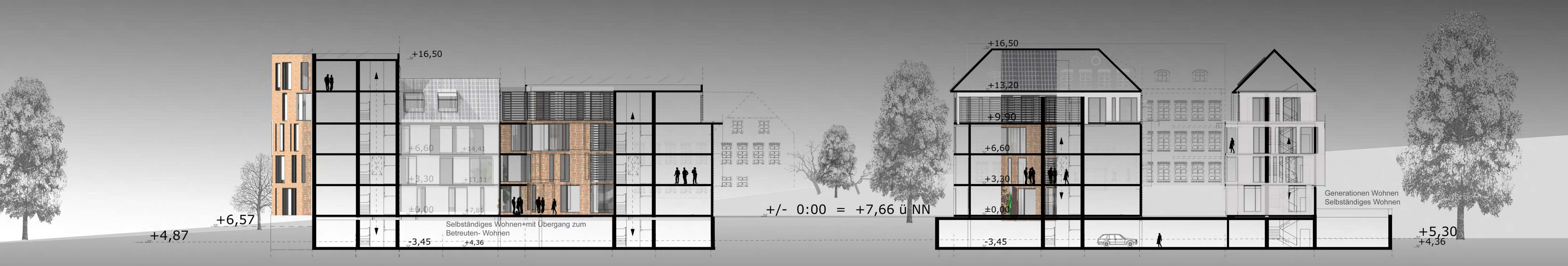
Schnitt- Ansicht M 1/200 Gartenstraße
