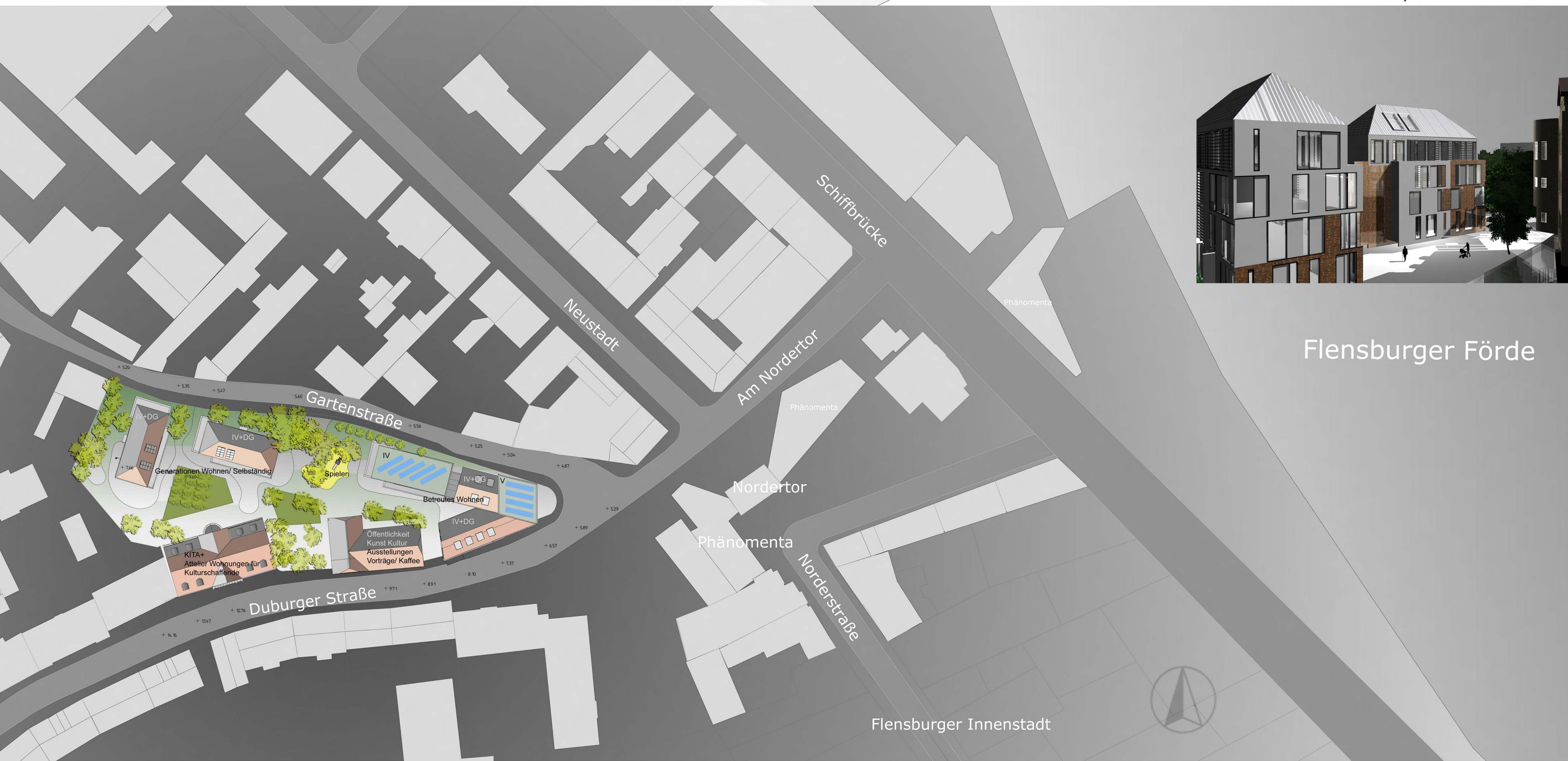
Lageplan M 1/500
